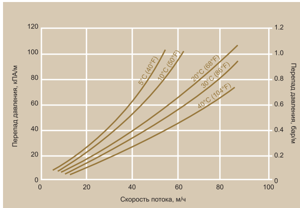
Перепад давления
