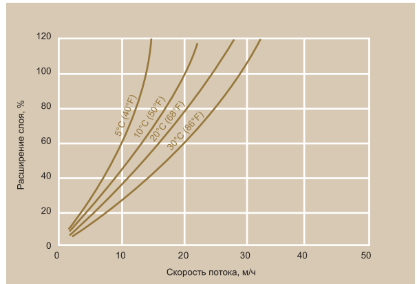
Расширение слоя при обратной промывке
